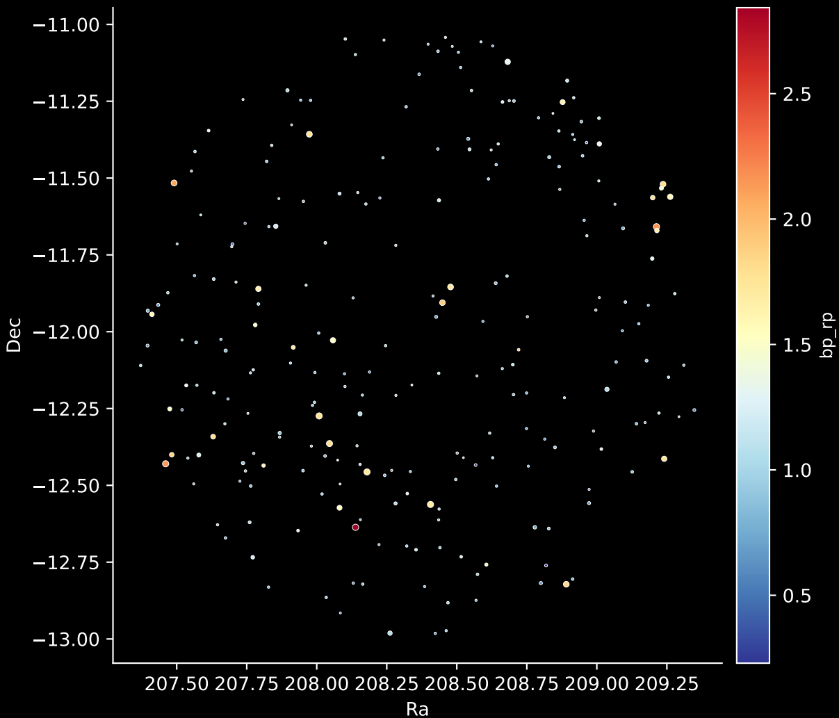
GALAH DR4 Field: [8828] Stars: 240
