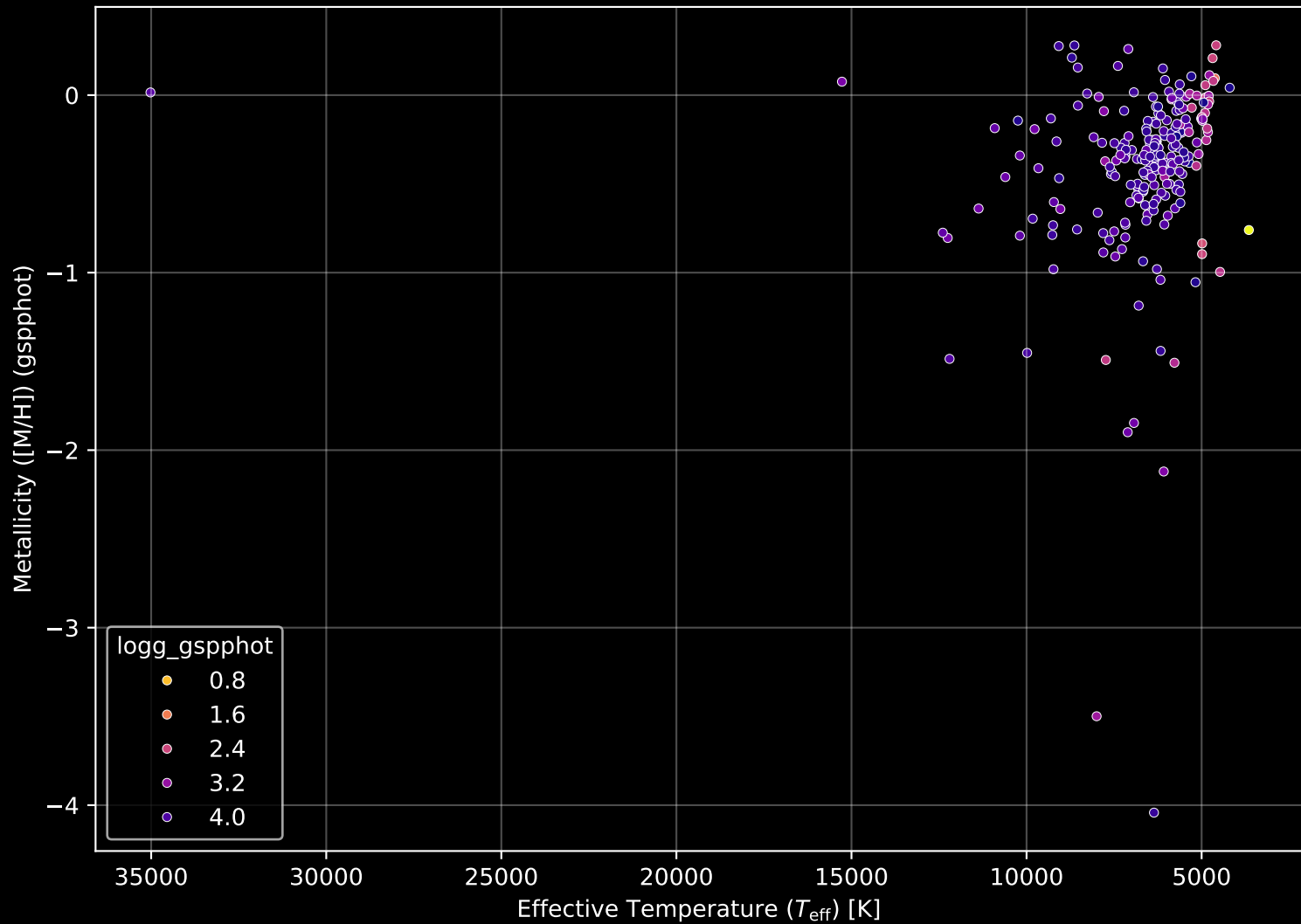
GALAH DR4 Field: [8828] Stellar Population Parameters (n= 240)
