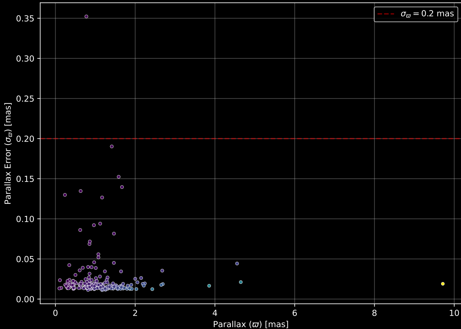
GALAH DR4 Field: [8828] Parallax Quality (n= 240)
