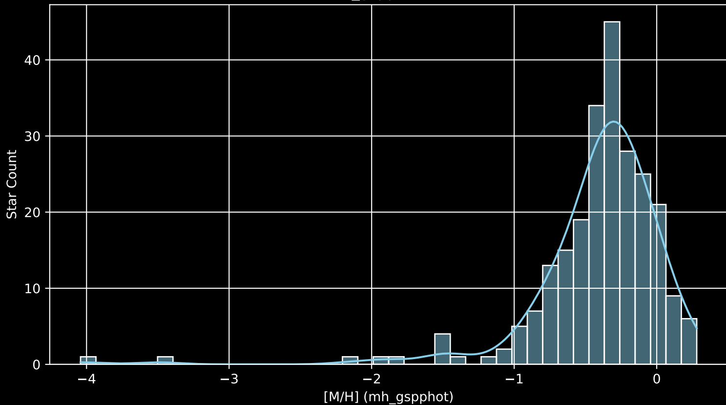
GALAH DR4 Field: [8828] [M/H] (mh_gspphot) (n= 240)
